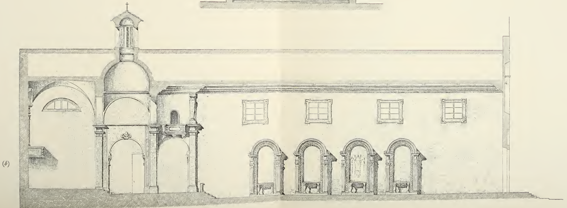
(a) Sezione trasversale. — (b) Sezione longitudinale.
